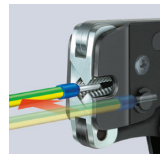
97 53 08: Införing av ändhylsor parallellt från sidan till 2,5 mm 2 t ex i trånga utrymmen
