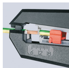
Exakt avisolering från 0,2 - 6,0 mm 2
